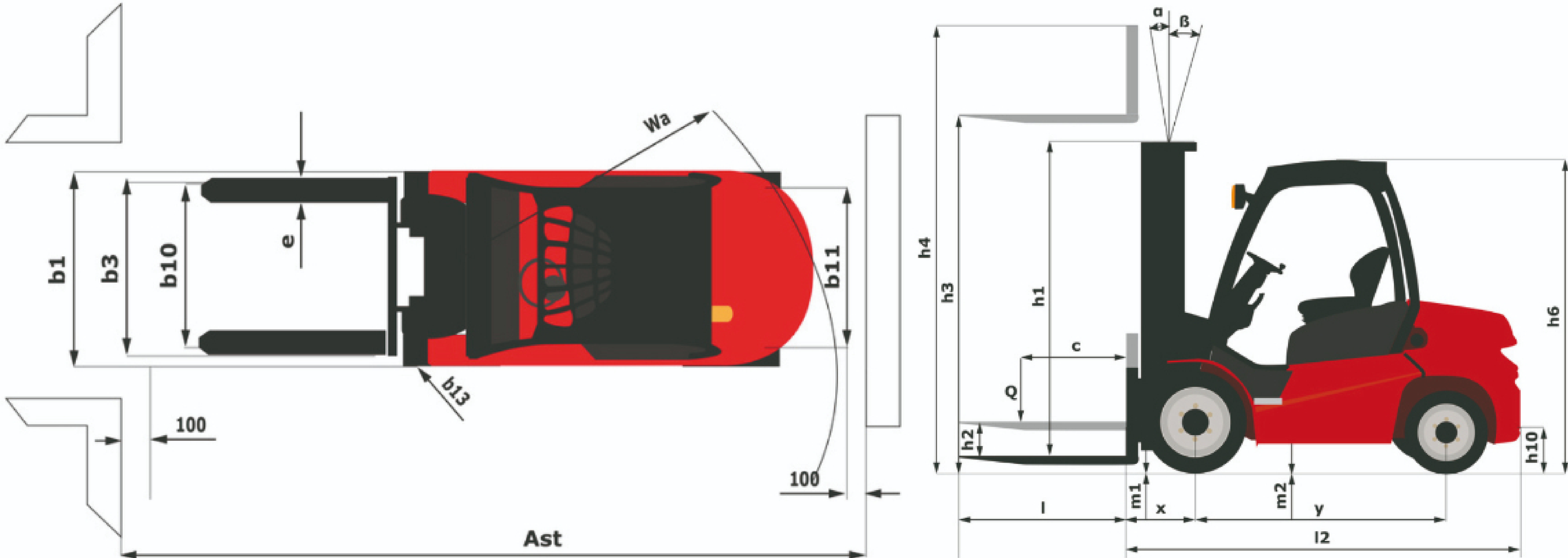
MI 25 D ST5 - Diagrama dimensional
